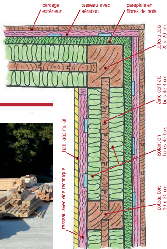
coupe d'un mur extérieur (vue du dessus)
